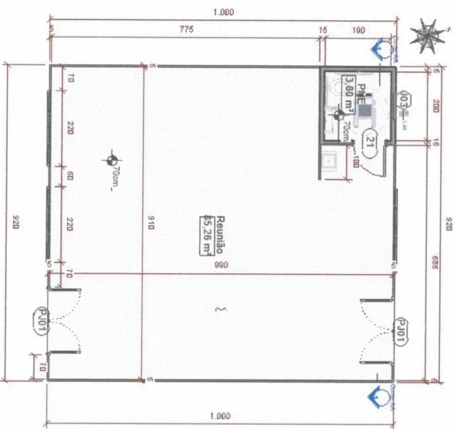
PLANTA BAIXA
