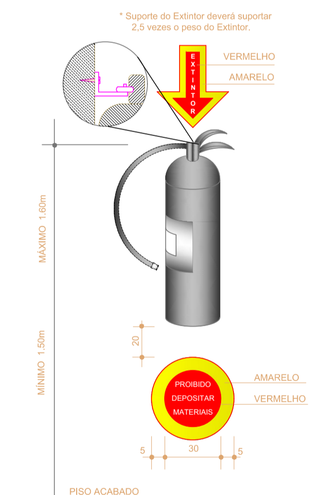
DETALHE EXTINTOR ESCALA 1/25
