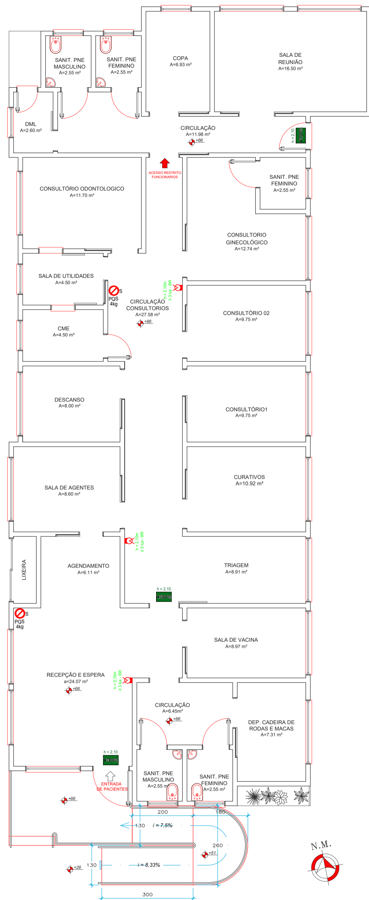
PLANTA BAIXA INSTALAÇÕES PREVENTIVAS CONTRA INCÊNDIO ÁREA = 254,57 m² ESCALA 1/75
