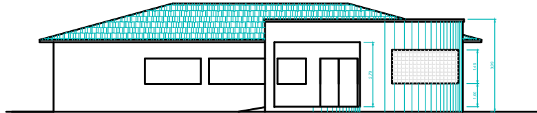
FACHADA PRINCIPAL Esc. 1:50
