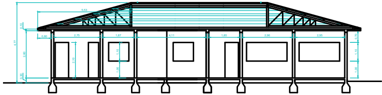
CORTE AA Esc. 1:50
