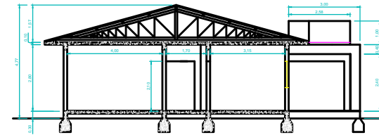
CORTE BB Esc. 1:50
